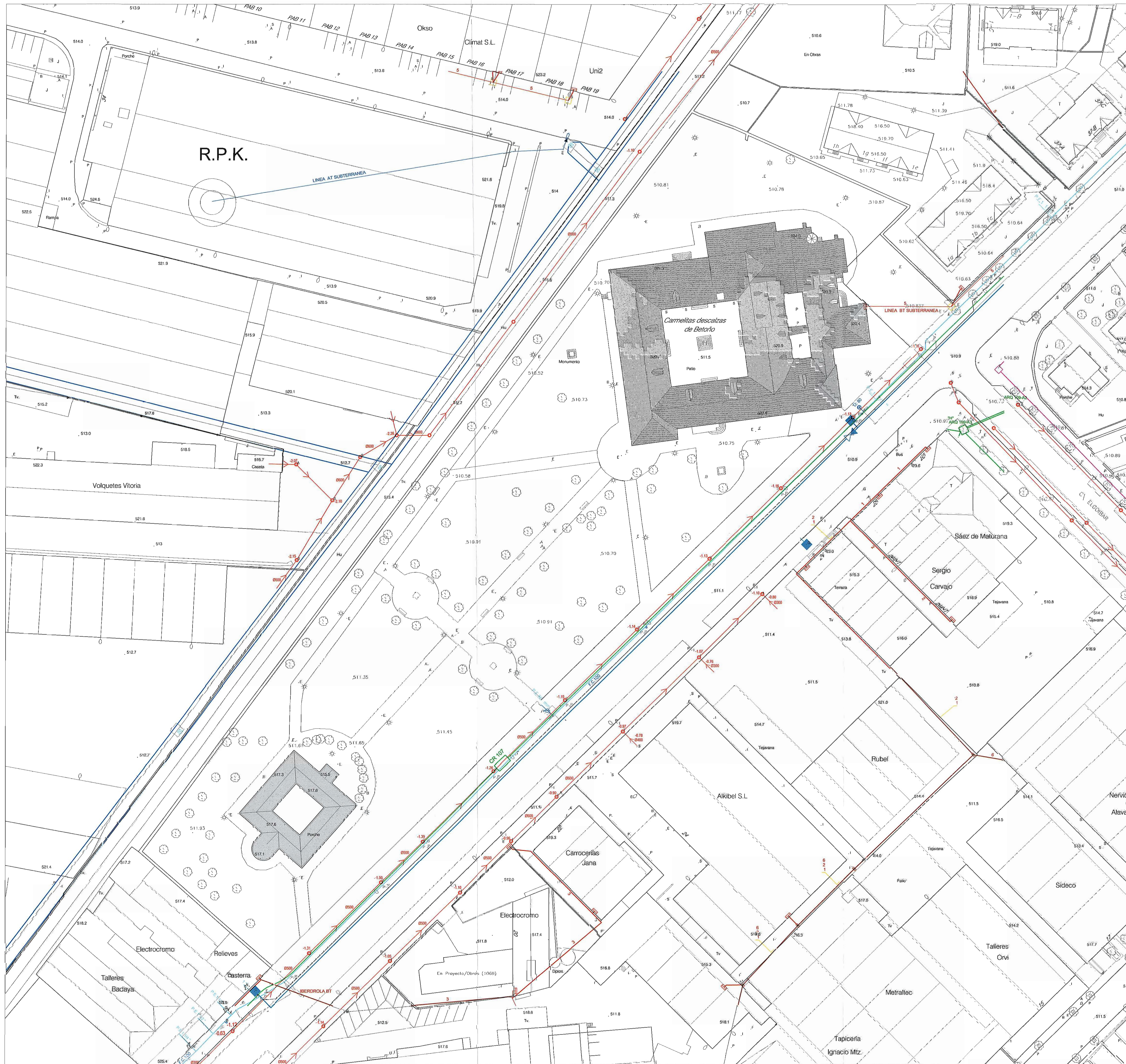
EMPLAZAMIENTO 1/500
