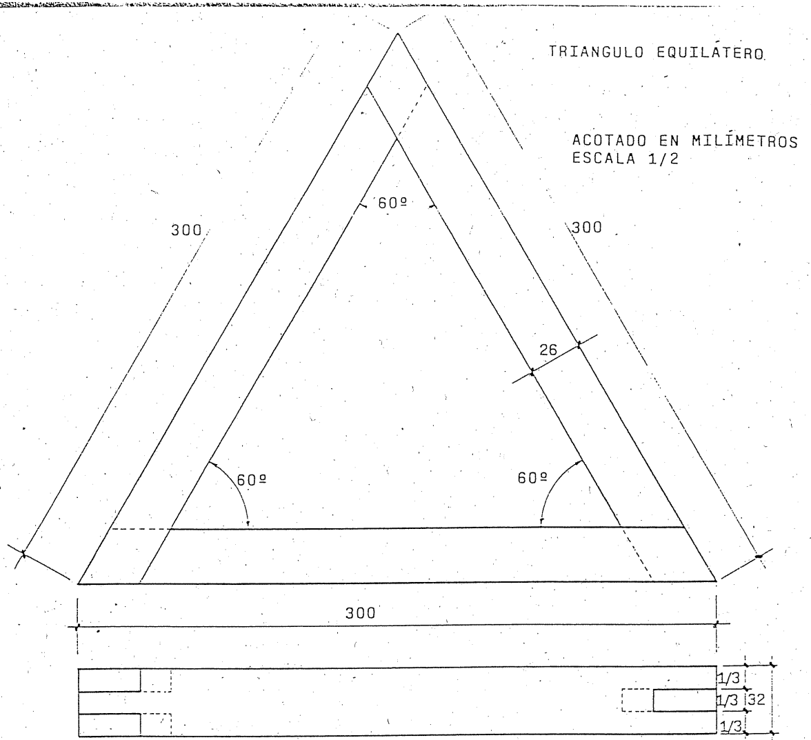
DETALLE DE ENSAMBLES EN HORQUILLA
