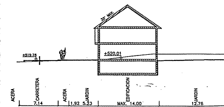
SECCION F-F
