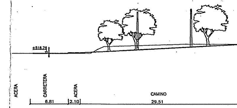
SECCION E-E
