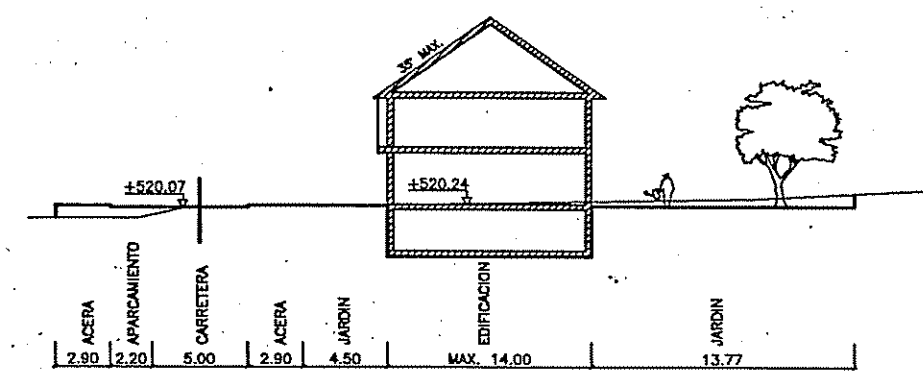
SECCION A-A
