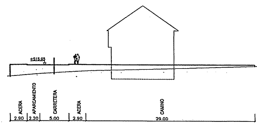
SECCION C-C
