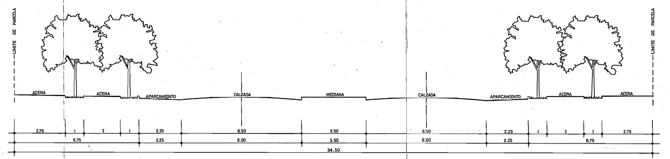
SECCION F-F (VL-7 TRAMO NORTE Y SUR)
