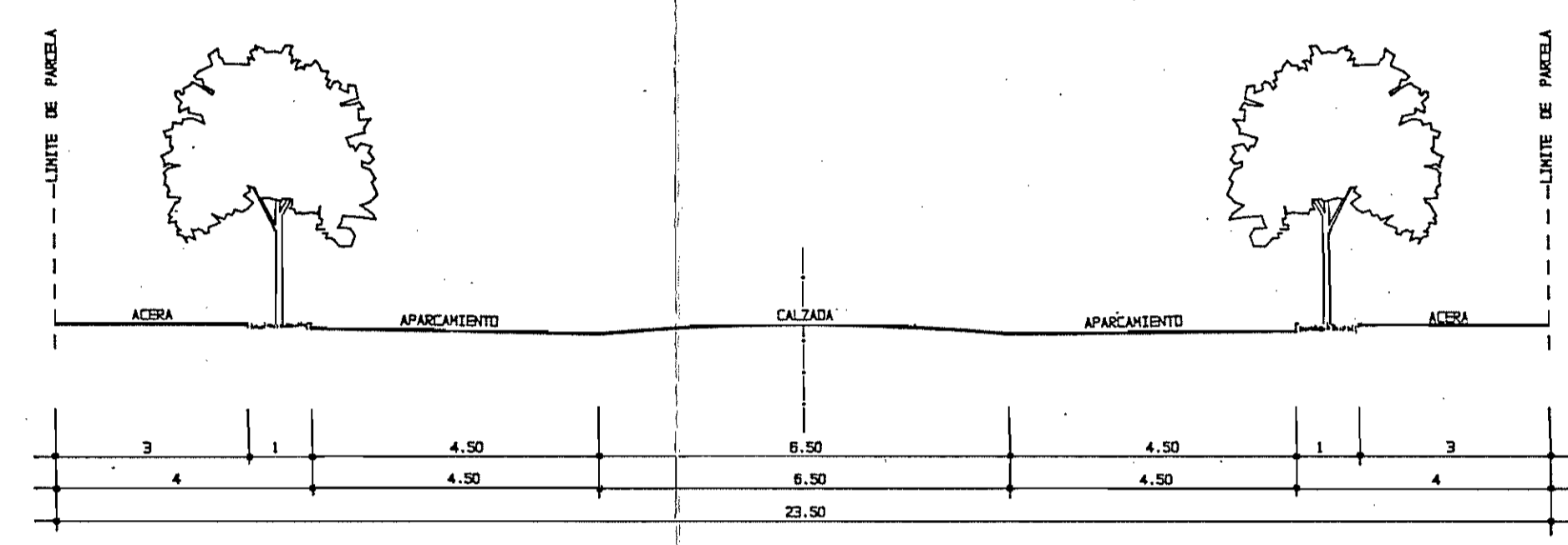
SECCION E-E (VL-6)
