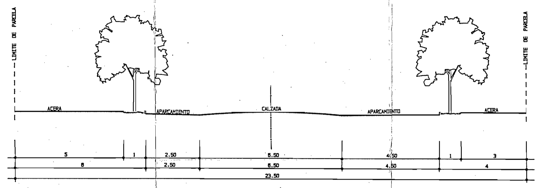
SECCION D-D (VL-5)
