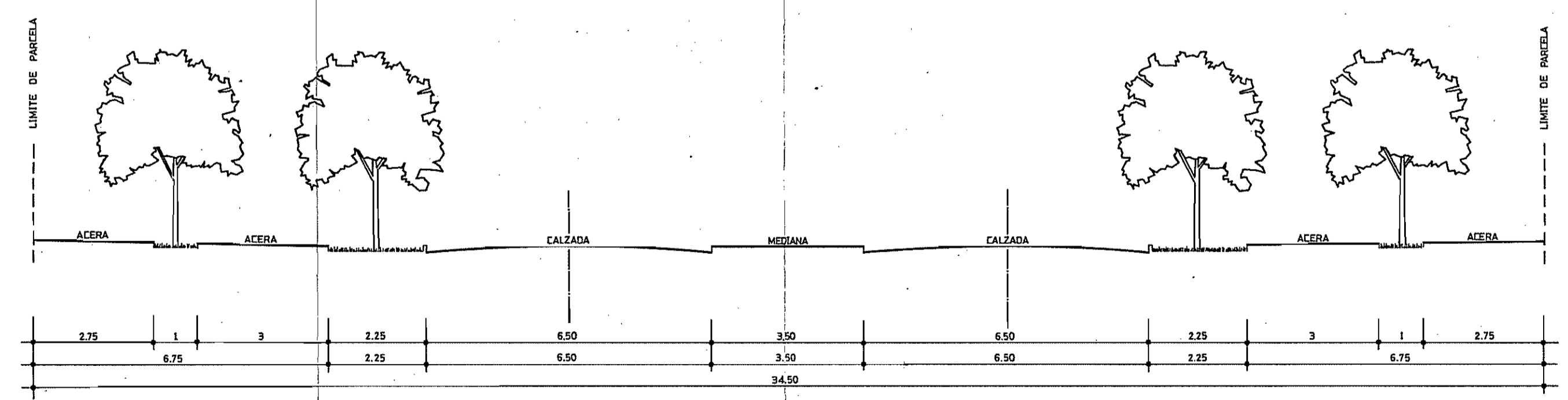
SECCION G-G (VL-7 TRAMO CENTRAL)
