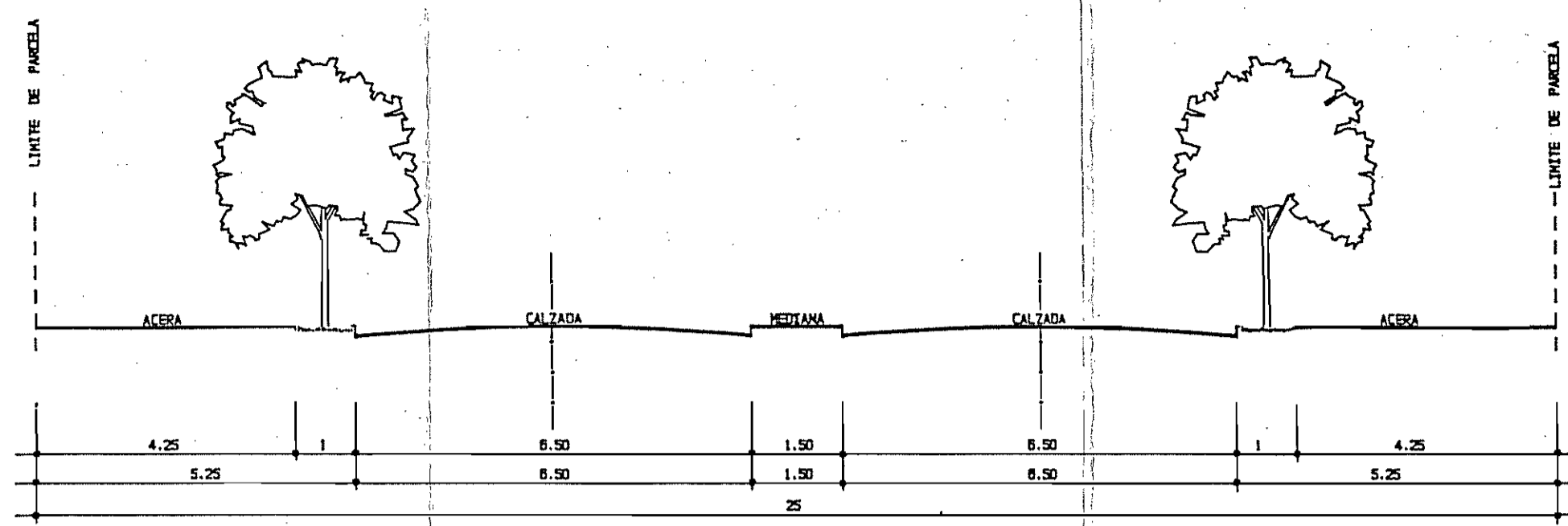
SECCION A-A (VL-1)
