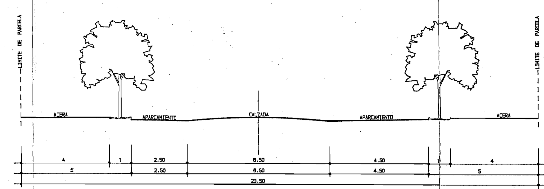
SECCION C-C (VL-3 VL-4)
