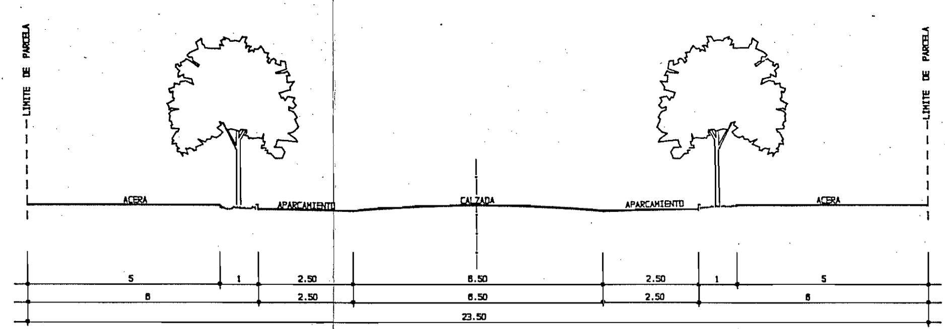
SECCION B-B (VL-2)
