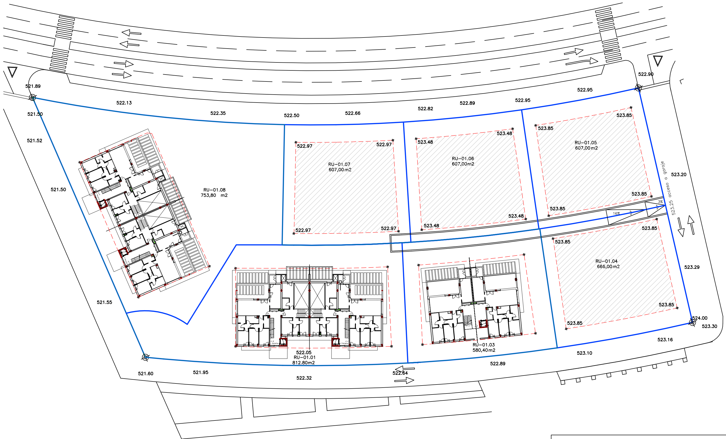
PLANTAS PRIMERAS: SUPERPOSICION AL AREA DE MOVIMIENTO DE EDIFICACION MAXIMA
