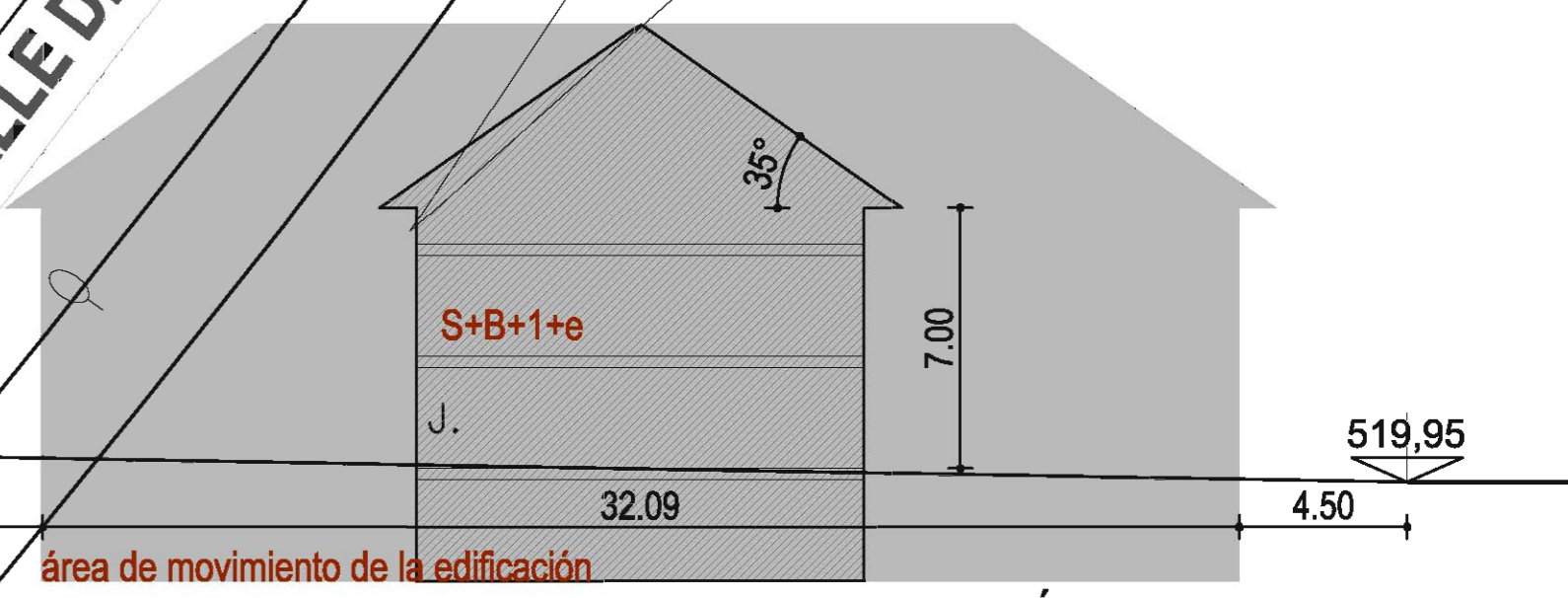
SECCIÓN TRANSVERSAL R.U. 04
