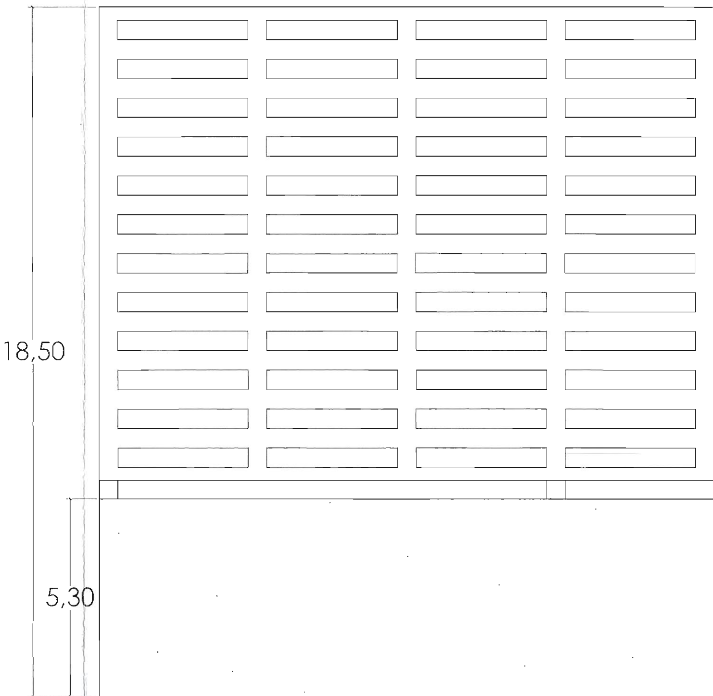
DETALLE DE CIERRE DE PARCELA COMPUESTO POR SÓCULO DE HORMIGÓN Y PANEL SUPERIOR DE CHAPA DE ACERO GALVANIZADO MOD. A 1200x DE CERRES AICAR (SISTEMA ANCAR 2)
